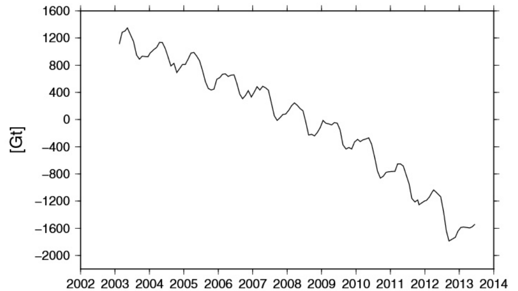
Abb. 4: Eisverlust von Grönland, berechnet aus GRACE Daten.
