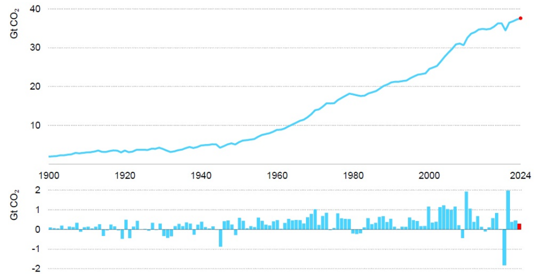
Abb. 29: Globale jährliche Emission von CO 2 aus Verbrennung fossiler Energieträger. Grafik aus [23].
