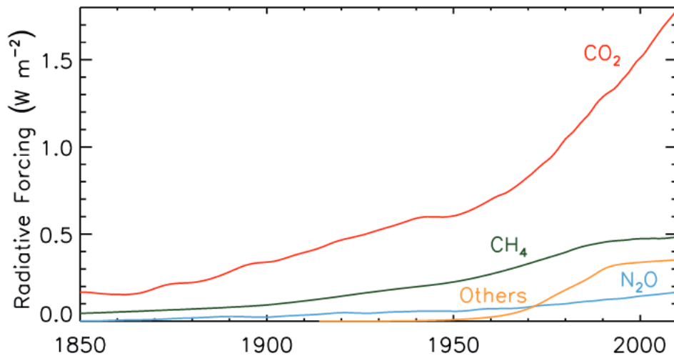
Abb. 22: Radiative Forcing der Treibhausgase. Grafik aus [5, chap. 8].
