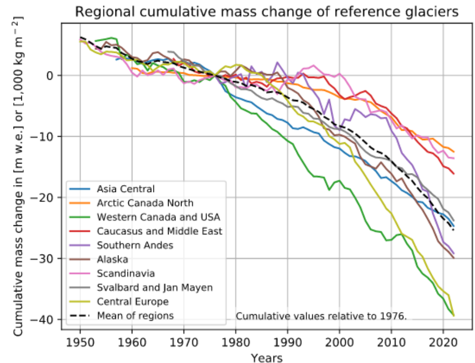
Abb. 2: Eisverlust von 41 Gebirgsgletschern. Grafik aus [2].
