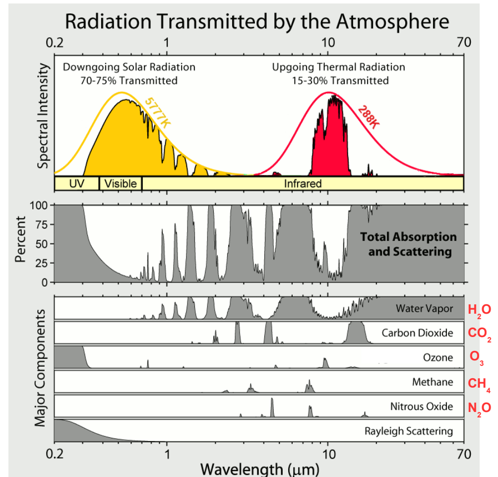
Abb. 21: Die Wirkung der Treibhausgase. Grafik aus [16].
