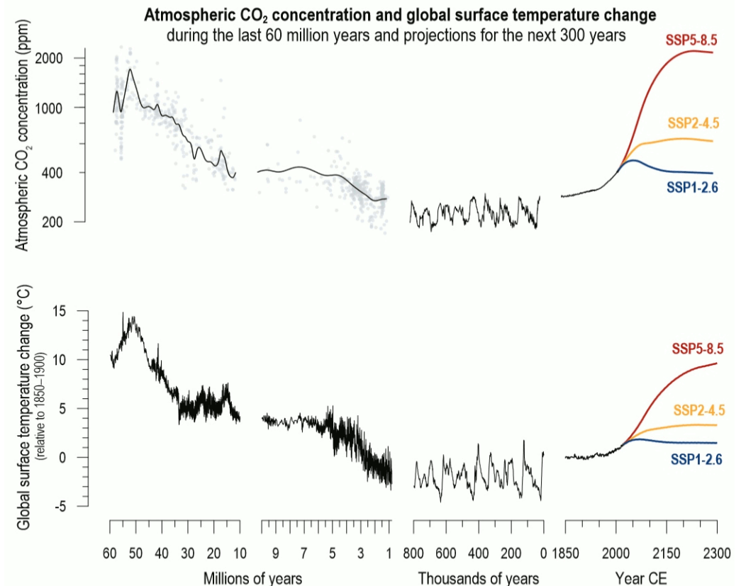
Abb. 33: Der Zusammenhang von CO 2 in der Atmosphäre und der Oberflächentemperatur der Erde. Grafik aus [17, fig. TS.1].
