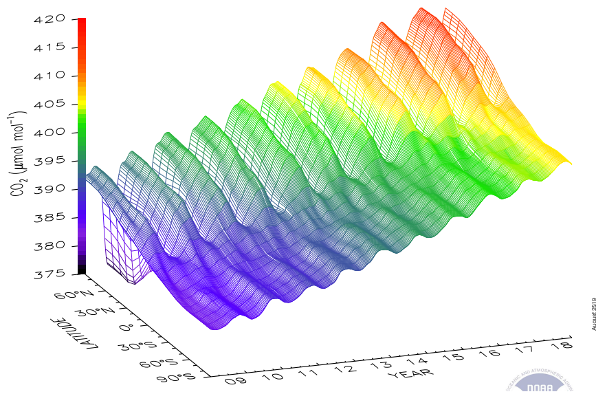
Abb. 14: Regionale Verteilung der \text{CO}_2 Konzentration in den Jahren 2009 bis 2018. Grafik aus [7].
