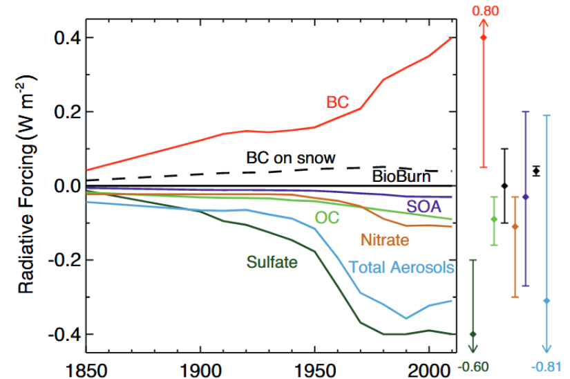
Abb. 23: Radiative Forcing der Aerosole. Grafik aus [5, chap. 8].
