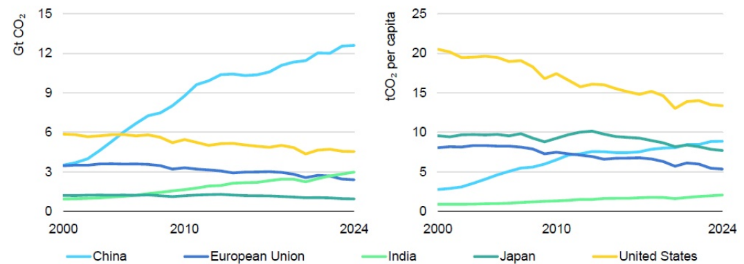
Abb. 30: Globale jährliche Emission von CO 2 pro Land (links) und pro Kopf (rechts) aus Verbrennung fossiler Energieträger. Grafik aus [23].
