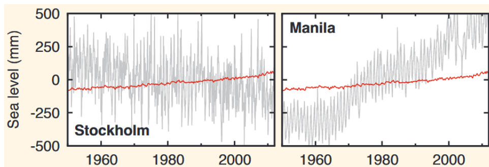
Abb. 8: Lokaler Pegel (grau) und Globaler Mittelwert (rot) des Meeresspiegels. Grafik aus [5, Chapter 13].
