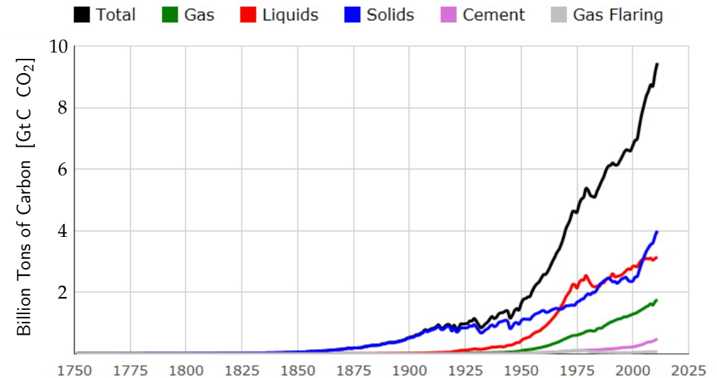
Abb. 28: Globale jährliche Emission von CO 2 aus Verbrennung fossiler Energieträger und Zementproduktion. Grafik aus [22].
