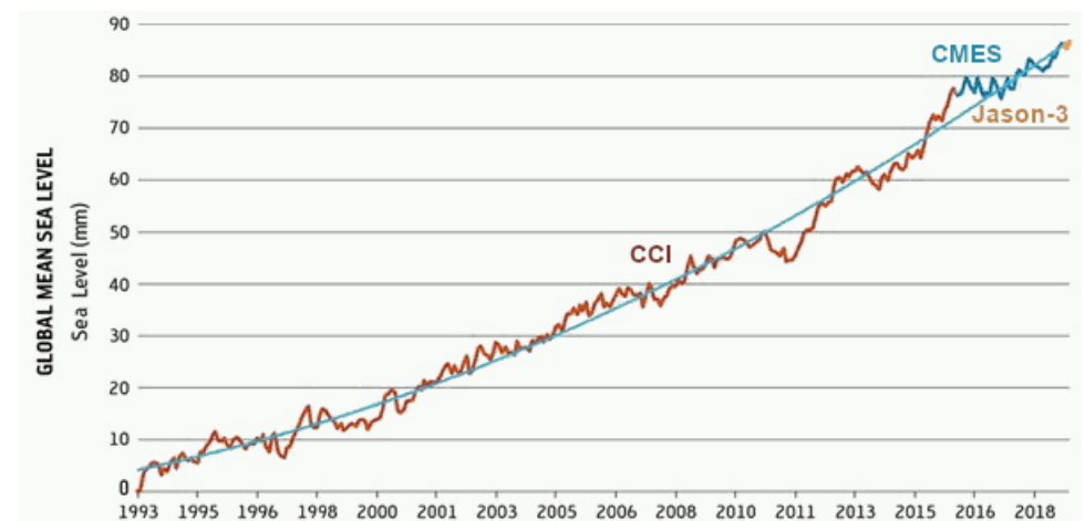
Abb. 9: Globales Mittel des Geozentrischen Meeresspiegels. Grafik aus [6].
