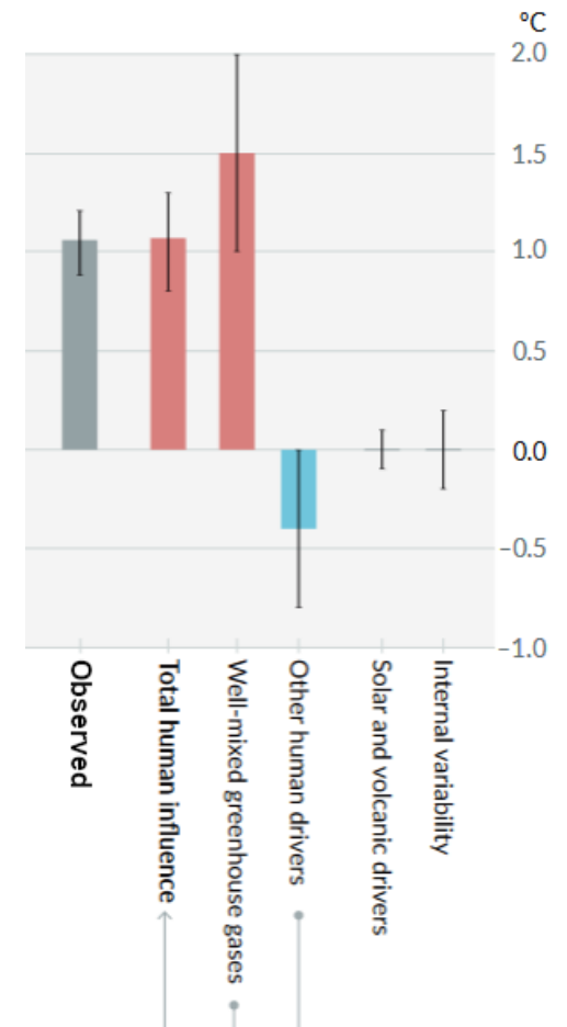
Abb. 26: Die Ursache der Erwärmung. Grafik aus [17, Fig. SPM.2].
