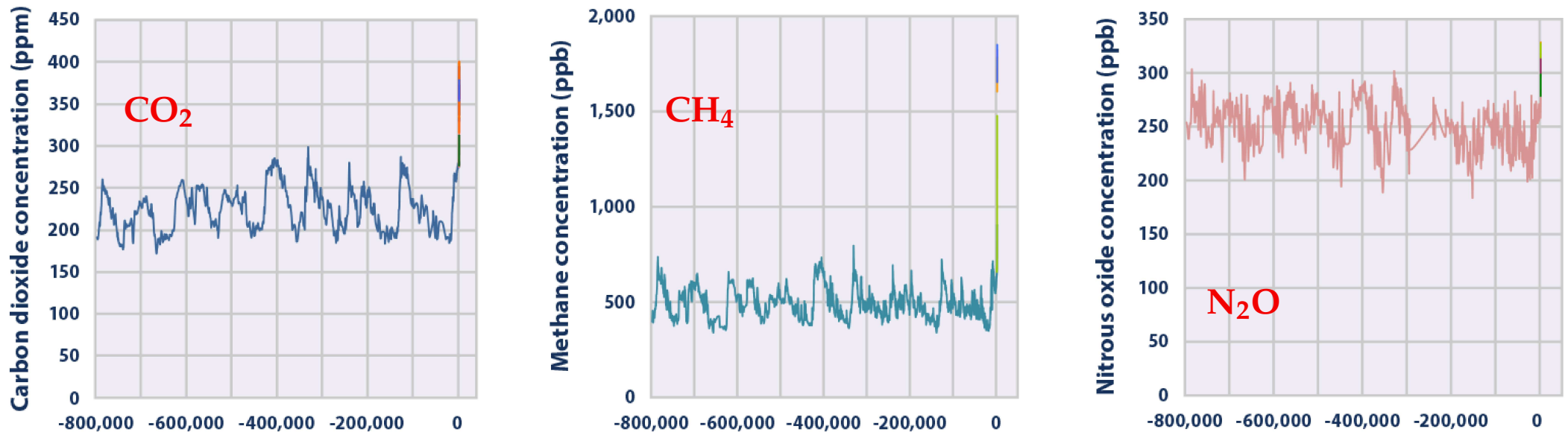
Abb. 17: Die Konzentrationen von \text{CO}_2 , \text{CH}_4 , und \text{N}_2\text{O} im Zeitraum -800 000 bis 2015. Die Messkurven bis 2015 sind jeweils ganz rechts in anderen Farben eingetragen. Grafik aus [8].
