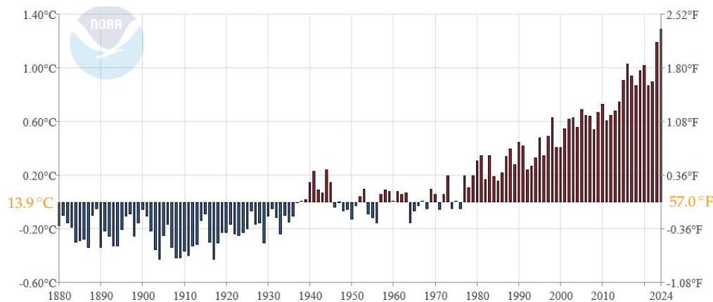
Abb. 1: Oberflächentemperatur, Globaler Jahresmittelwert von Meer und Land. Grafik aus [1].
