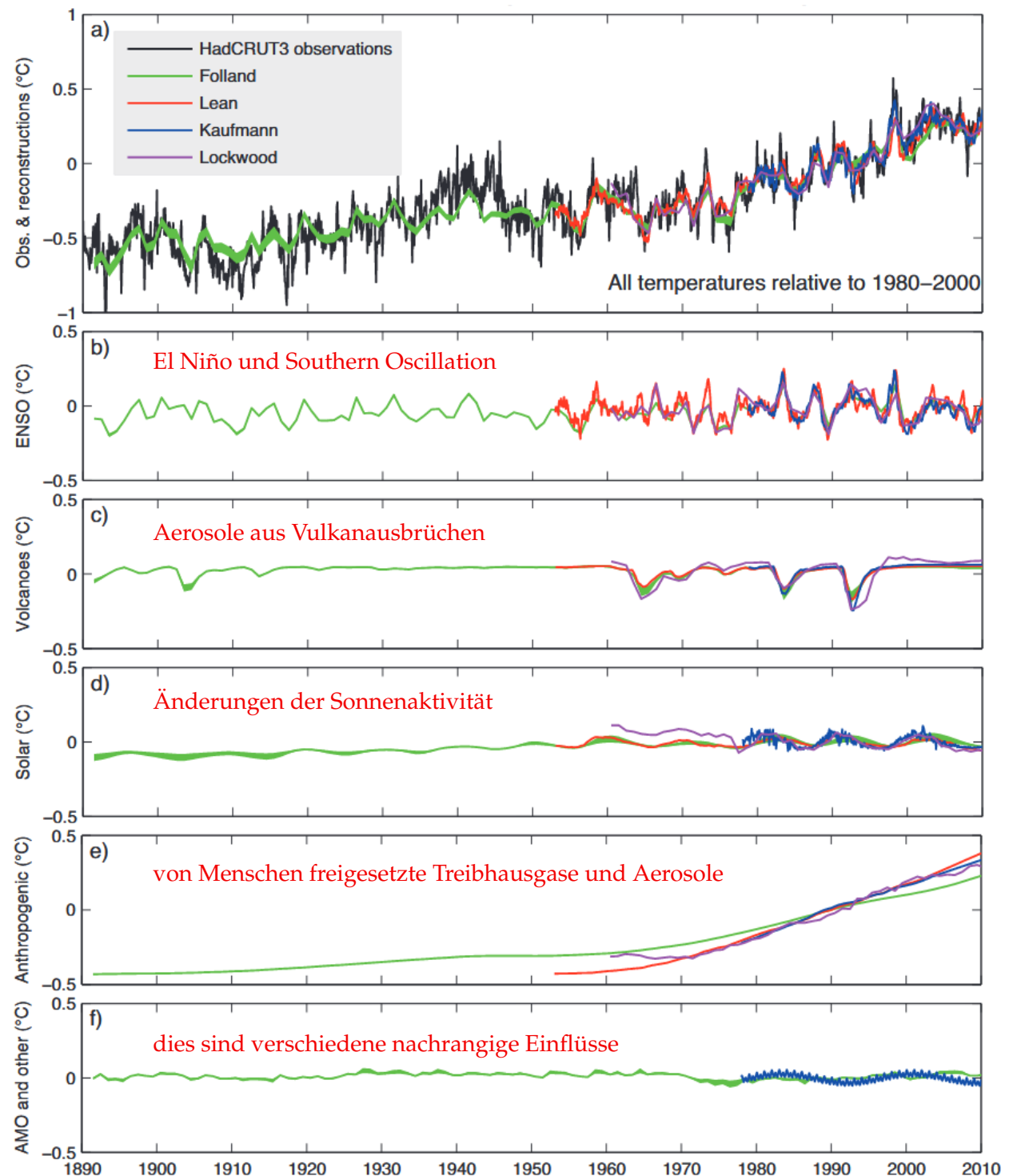
Abb. 25: Einfluss verschiedener Faktoren auf die Temperatur, berechnet mit vier verschiedenen Klimamodellen. Grafik aus [5, chap. 10].
