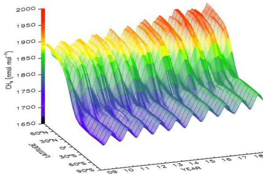
Abb. 15: Regionale Verteilung der \text{CH}_4 Konzentration in den Jahren 2009 bis 2018. Grafik aus [7].
