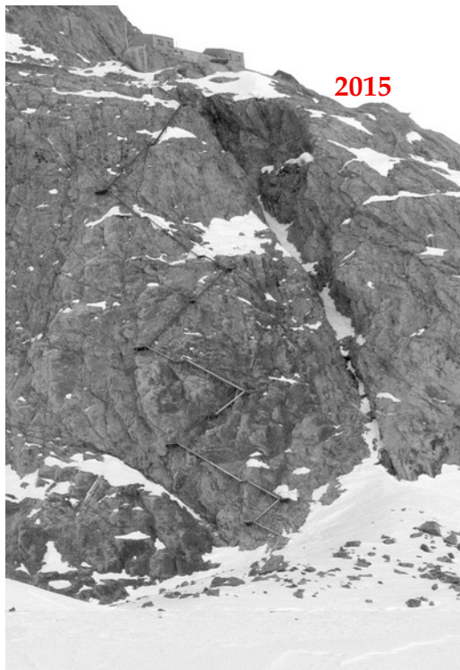
Abb. 3: Die Konkordiahütte über dem Aletschgletscher (Berner Alpen, Schweiz) gegen 1880 and im März 2015.
