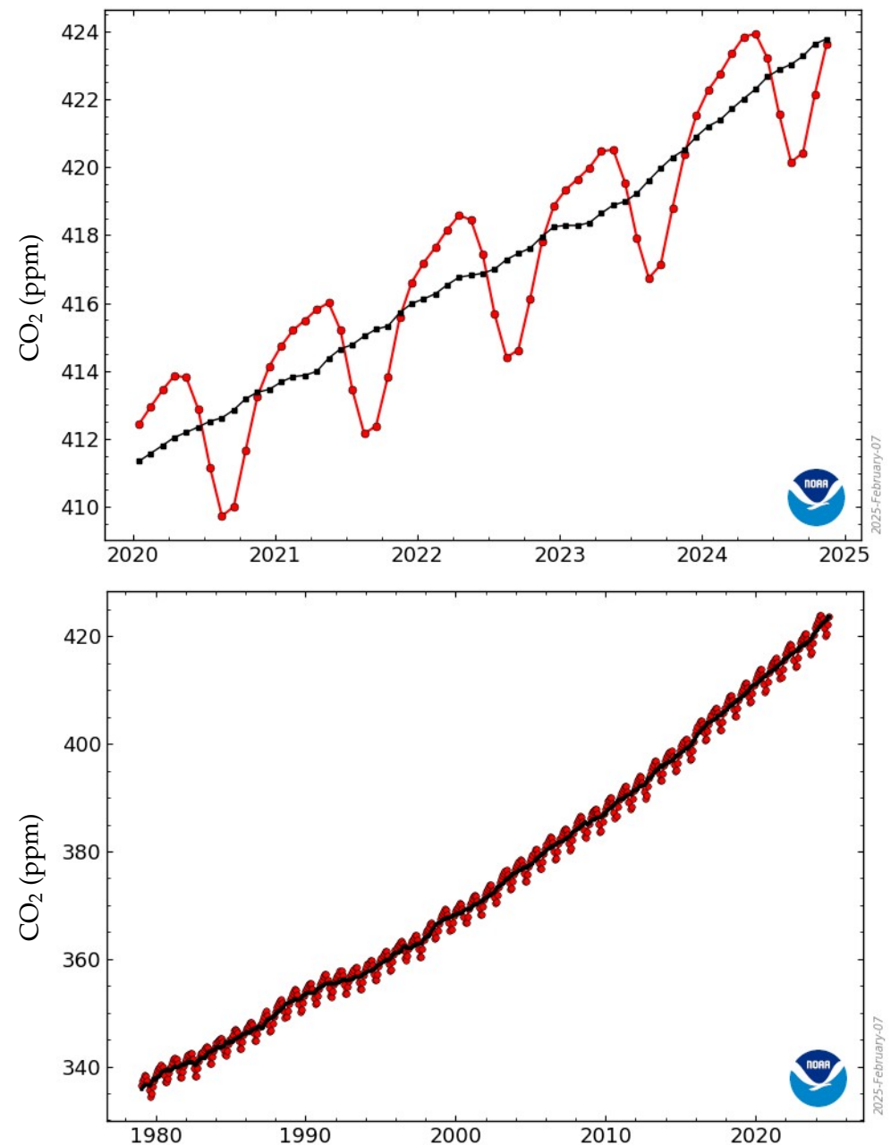
Abb. 10: Globaler Mittelwert der CO 2 Konzentration seit 2020 (oben) und seit 1980 (unten). Grafik aus [7].
