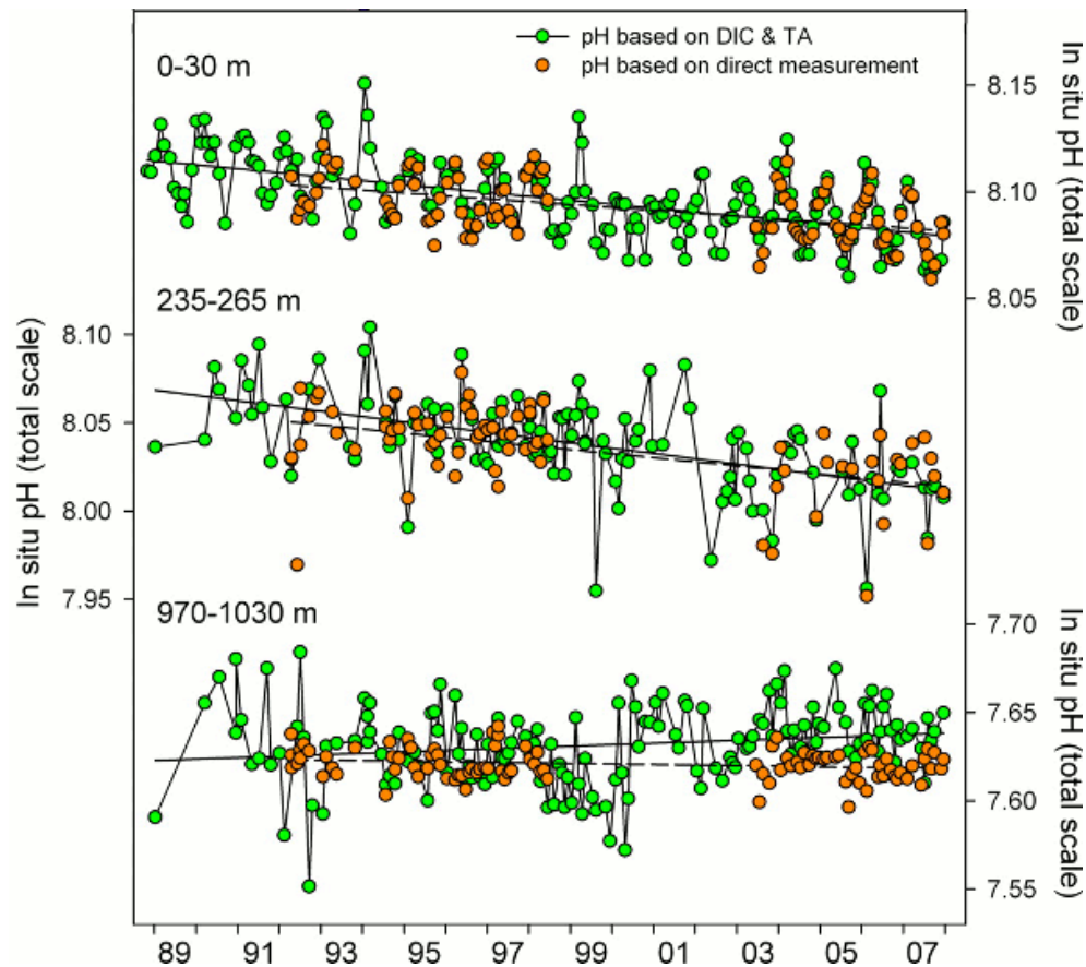
Abb. 18: pH-Werte in unterschiedlichen Meerestiefen. Station ALOHA, 1988–2007. Grafik aus [9].
