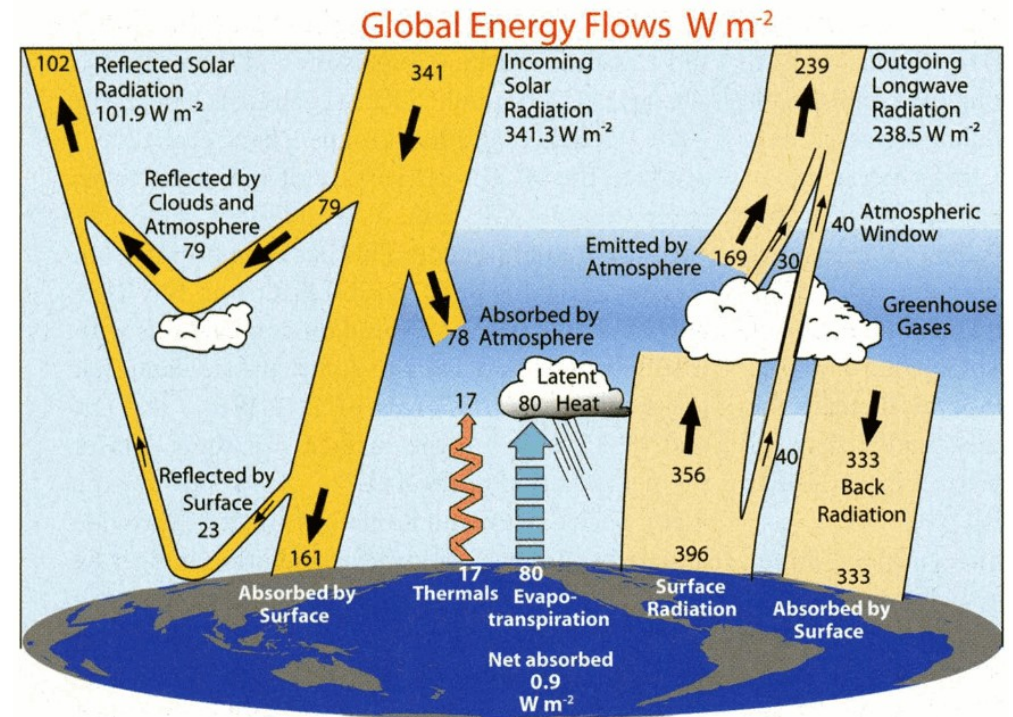
Abb. 19: Die Strahlungsbilanz der Erde. Grafik aus [13].
